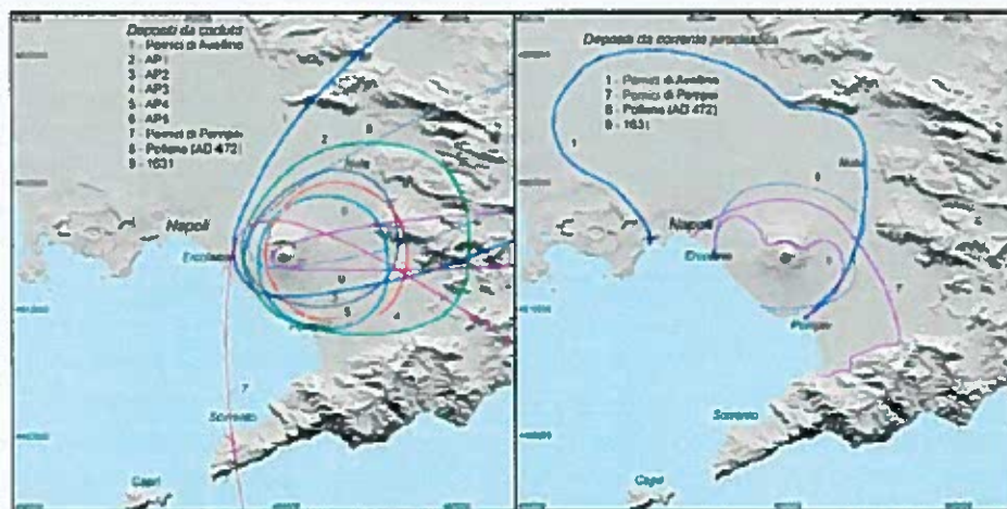
Distribuzione dei depositi delle eruzioni principali degli ultimi 4000 anni. Le linee indicano le isopache di 10 cm di spessore dei depositi da caduta (a sinistra) e l'area coperta dai depositi da corrente piroclastica (a destra) da Di Vito et al, 2013b
