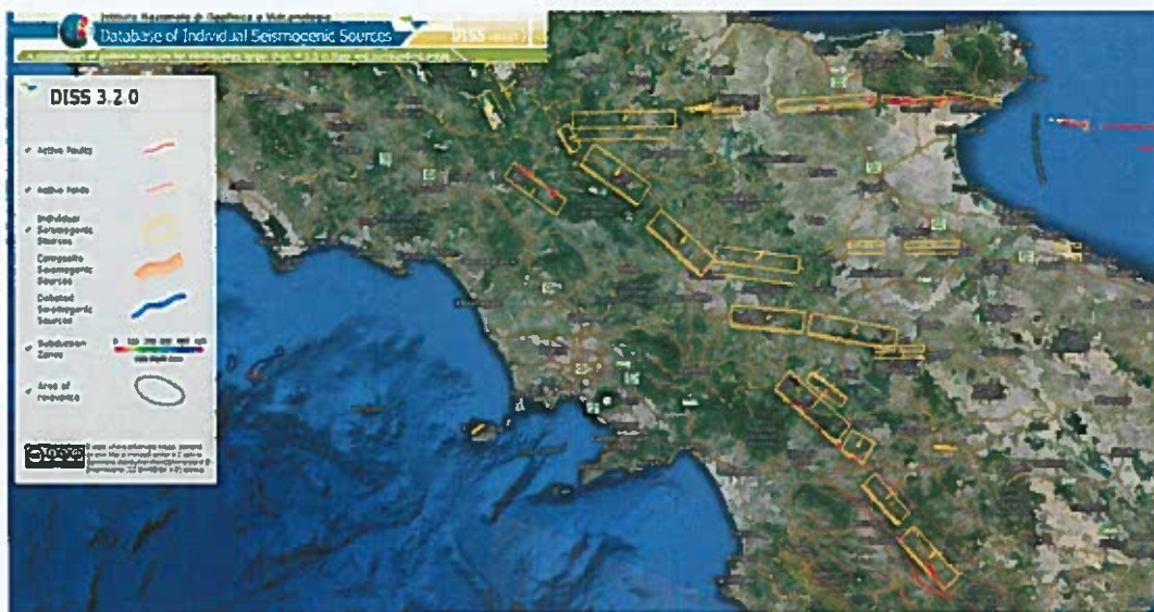
Sorgenti sismogenetiche - Fonte DISS (Database of Individual Seismogenic Sources)
