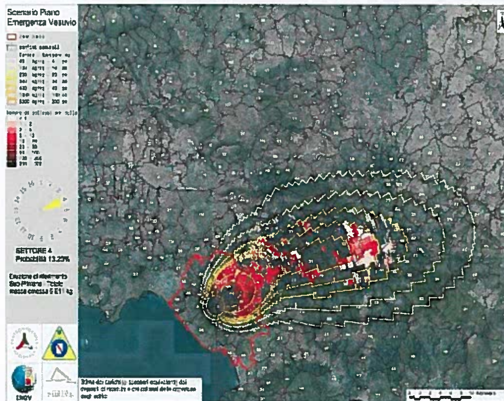
Scenario di riferimento – eruzione del 1631
