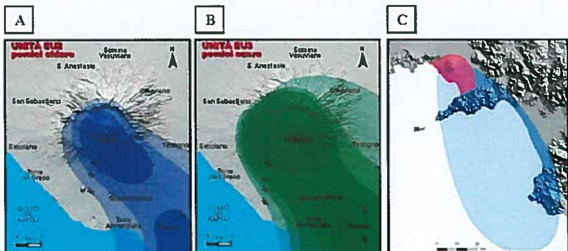
Carta delle isopache per i depositi delle Unità EU2 (deposito da caduta costituito da pomici di colore chiaro che termina con livelli cineritici da flusso) ed EU3 (pomici da caduta di colore grigio scuro, con intercalazioni di depositi cineritici da flusso generatisi da parziali collassi della colonna eruttiva) (da Sturasson et al.1985 – modificato) C: distribuzione areale dei depositi da caduta (in azzurro) e dei depositi da flusso piroclastico (in rosso) dell'eruzione del 79 d. c.
