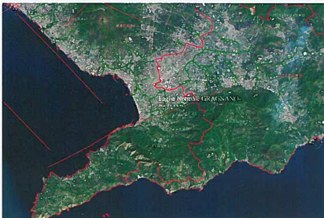
Cartografia faglie capaci estratta da banca –dati Ispra
