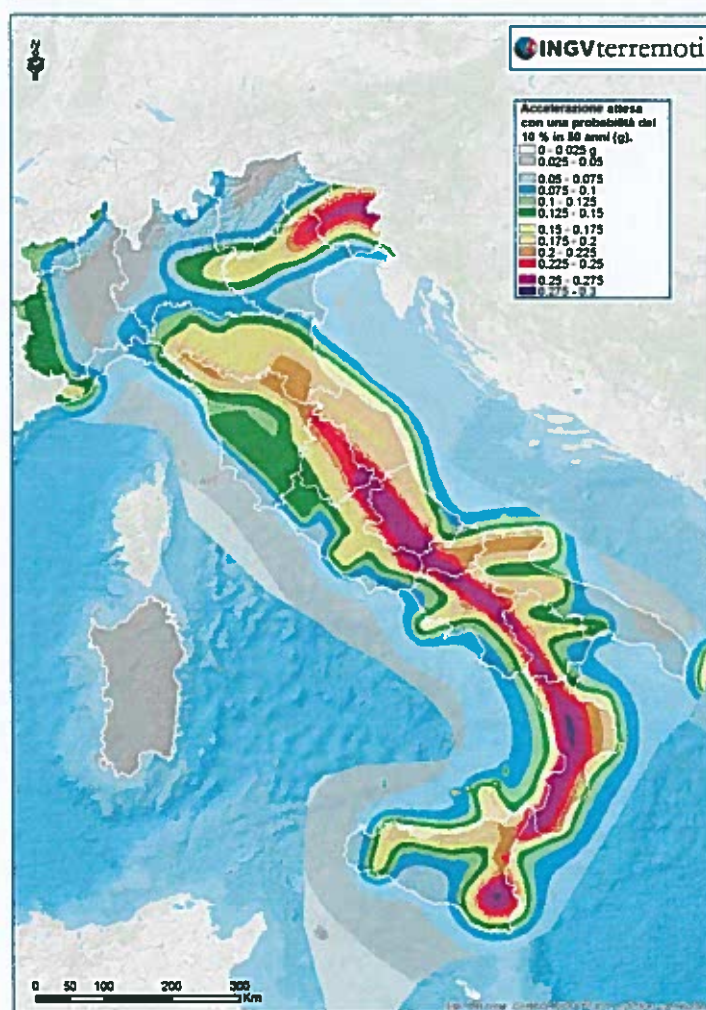
Accelerazioni di picco aventi il 10% di probabilità di essere superate in un tempo di interesse di 50 anni per il territorio italiano.
